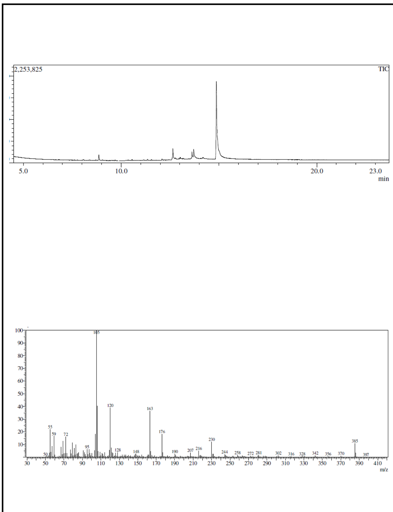
Espectro 40 – GC-MS (70 eV) da \alpha -metil- N -benzil-9- Z -octadecenamida (67c).
