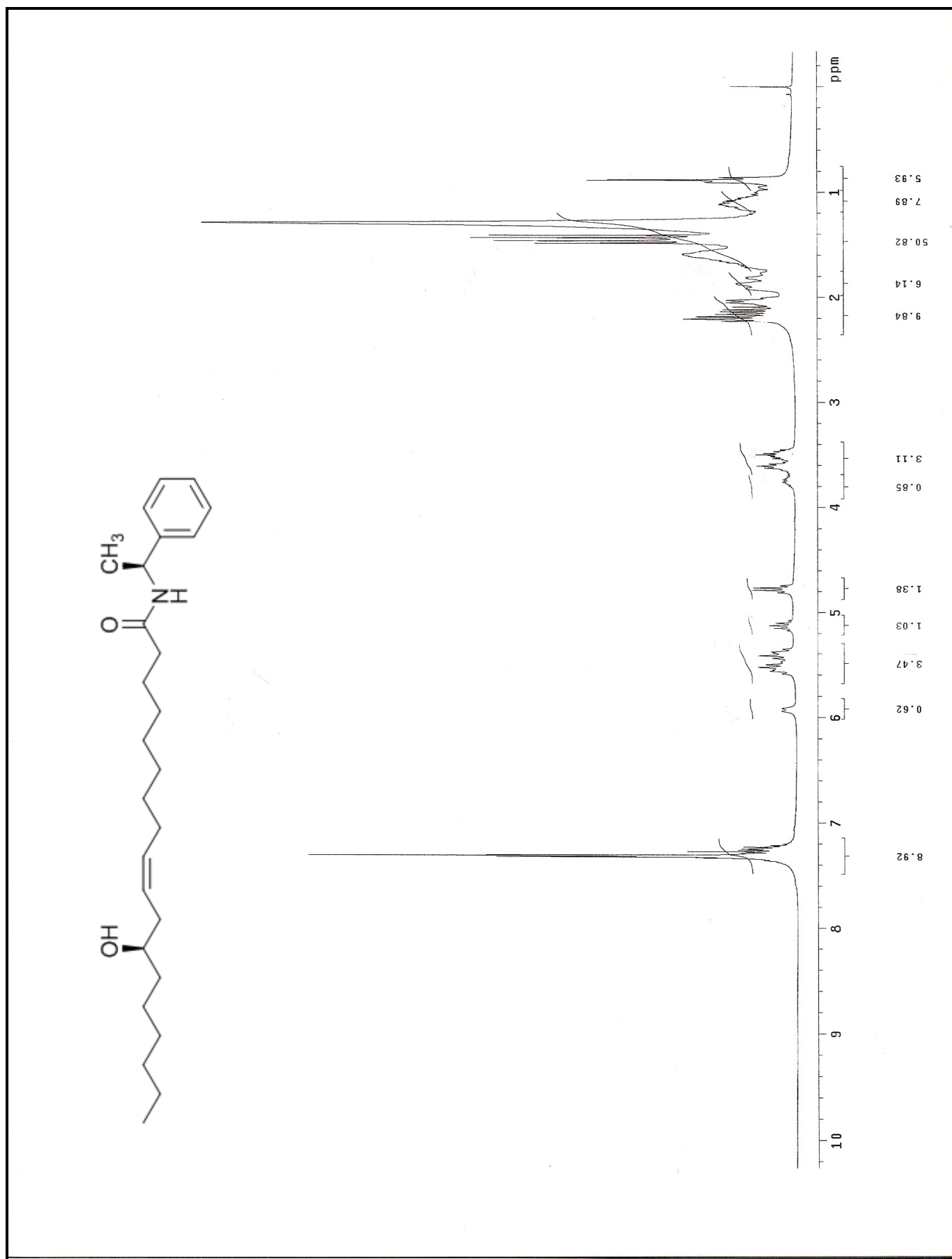
Espectro 44 – RMN ^1\text{H} (300 Hz, \text{CDCl}_3 ) da ( R/S )- \alpha -metil- N -benzil-12-hidróxi-9- Z -octadecenamida ( 67d ).
