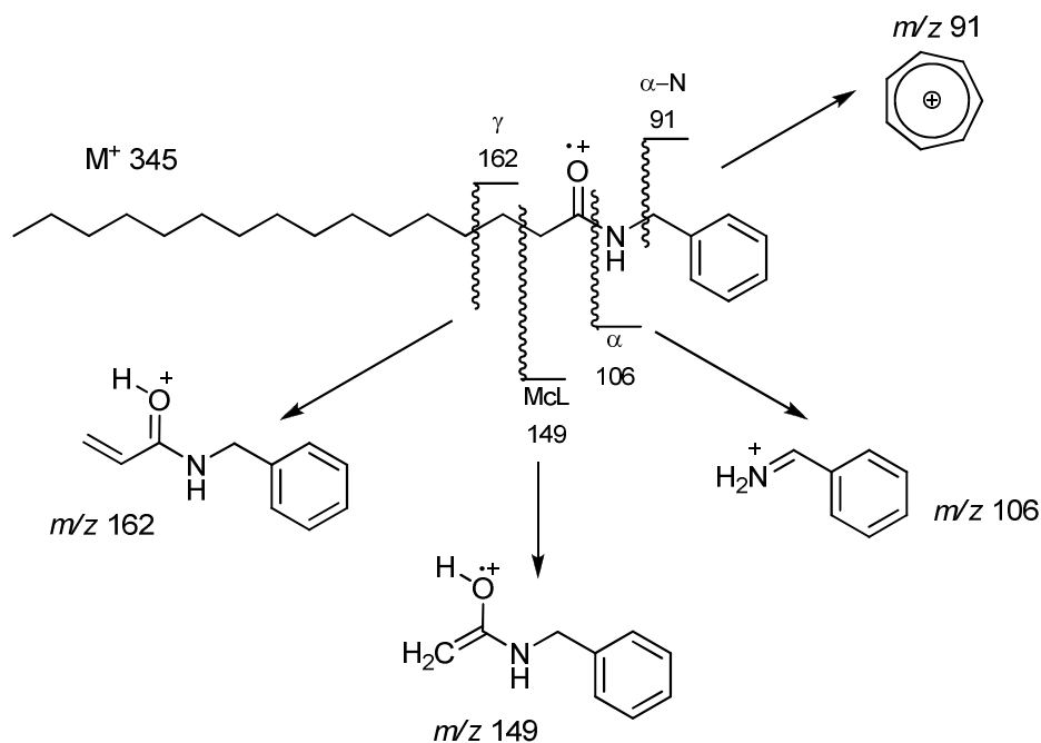
Figura 30 - Proposta de fragmentação para 66a .
