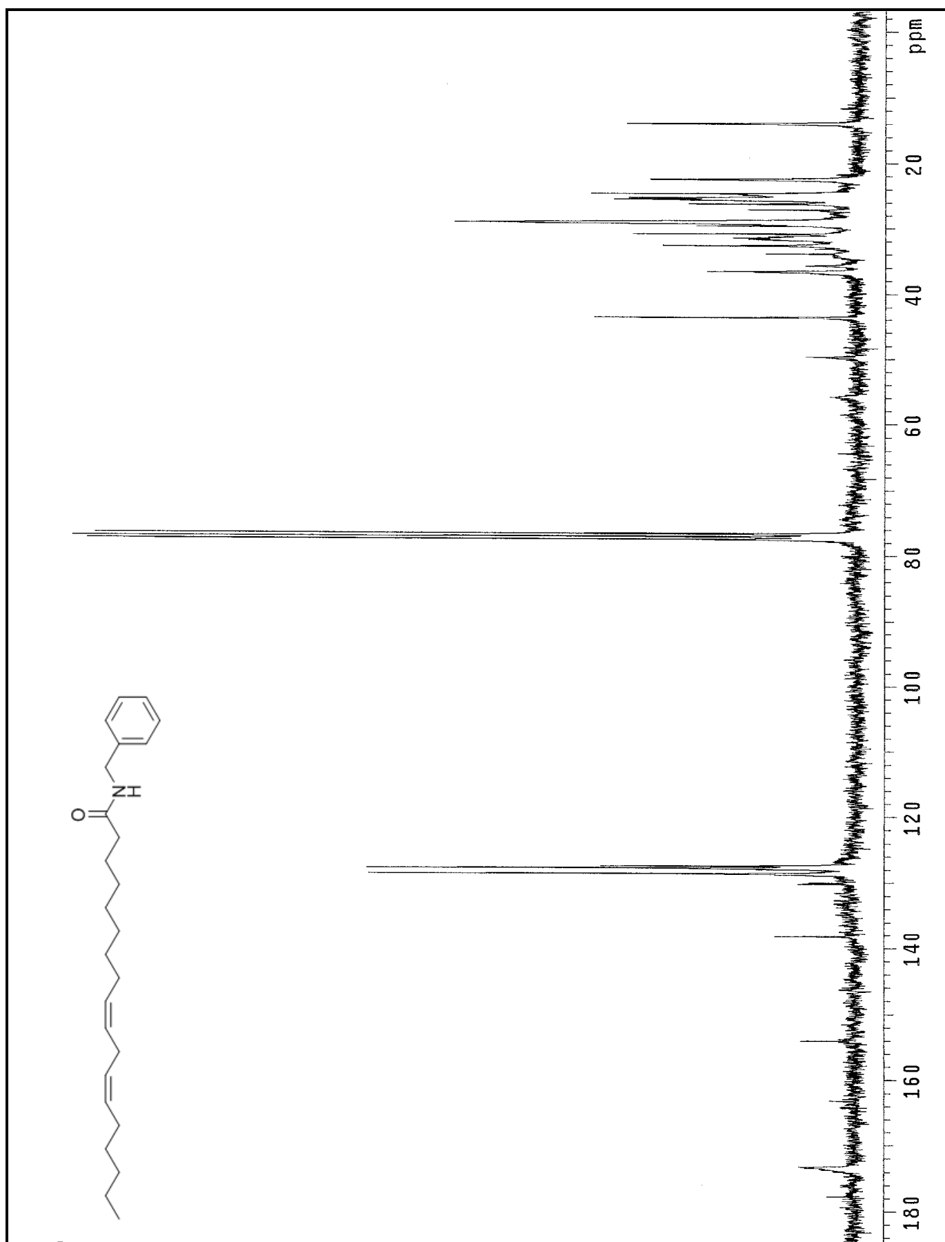
Espectro 26 – RMN ^{13}\text{C} (75 Hz, \text{CDCl}_3 ) da N -benzil-9,12- Z -octadidecenamida ( 66e ).
