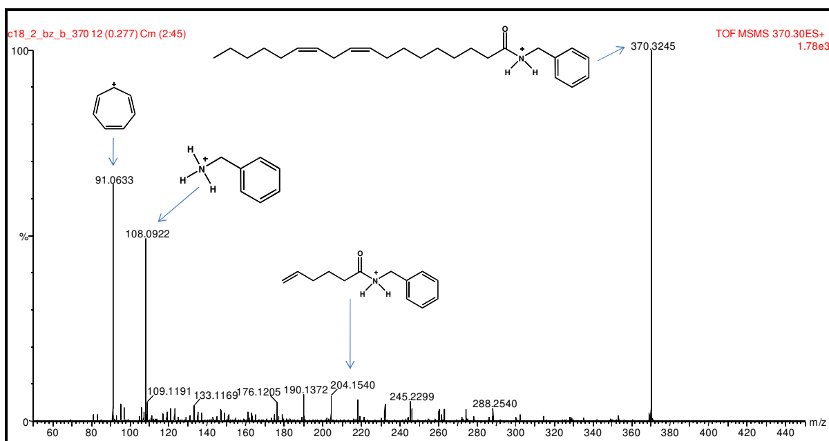
Figura 31 – Espectro de massas ESI-(+)-MS/MS da N-benzil-9-Z-10-Z-octadecenamida 66e .
