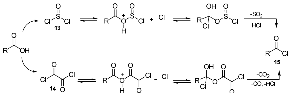
Esquema 3 - Mecanismo formação cloreto de acila utilizando cloreto de tionila 13 ou cloreto de oxalila 14 .
