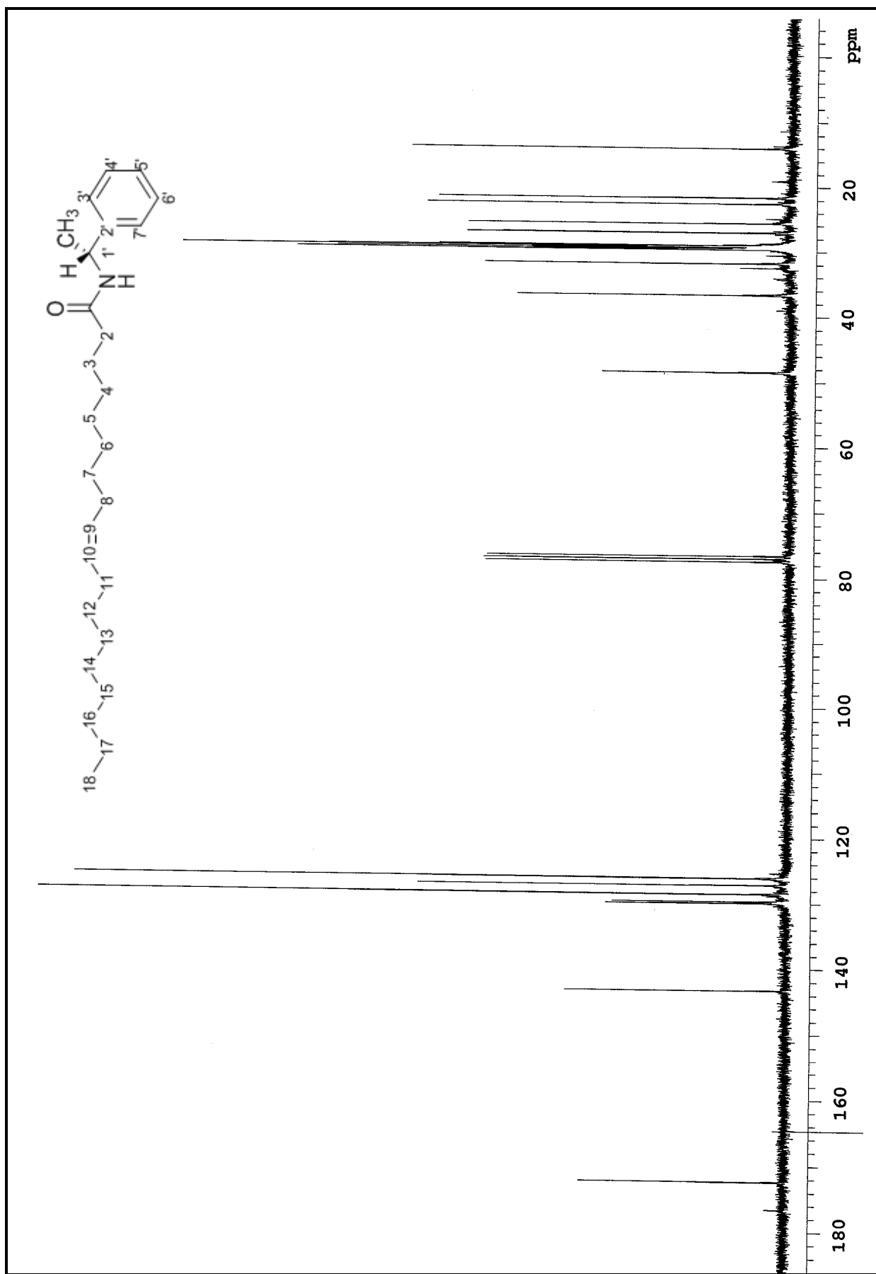
Figura 24 - Espectro RMN ^{13}\text{C} (75 MHz), para (R)-(+)-oleilmetilbenzilamida (R)-67c em \text{CDCl}_3 .
