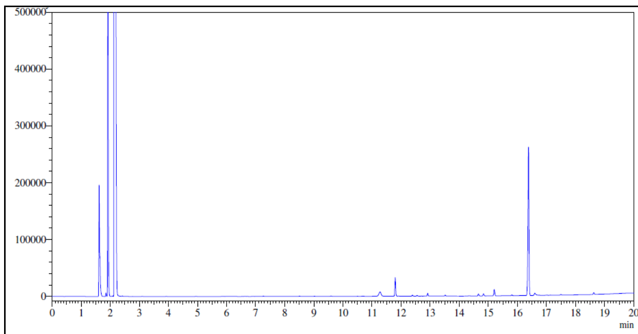
Cromatograma 2 – Estearato de metila 63b.
