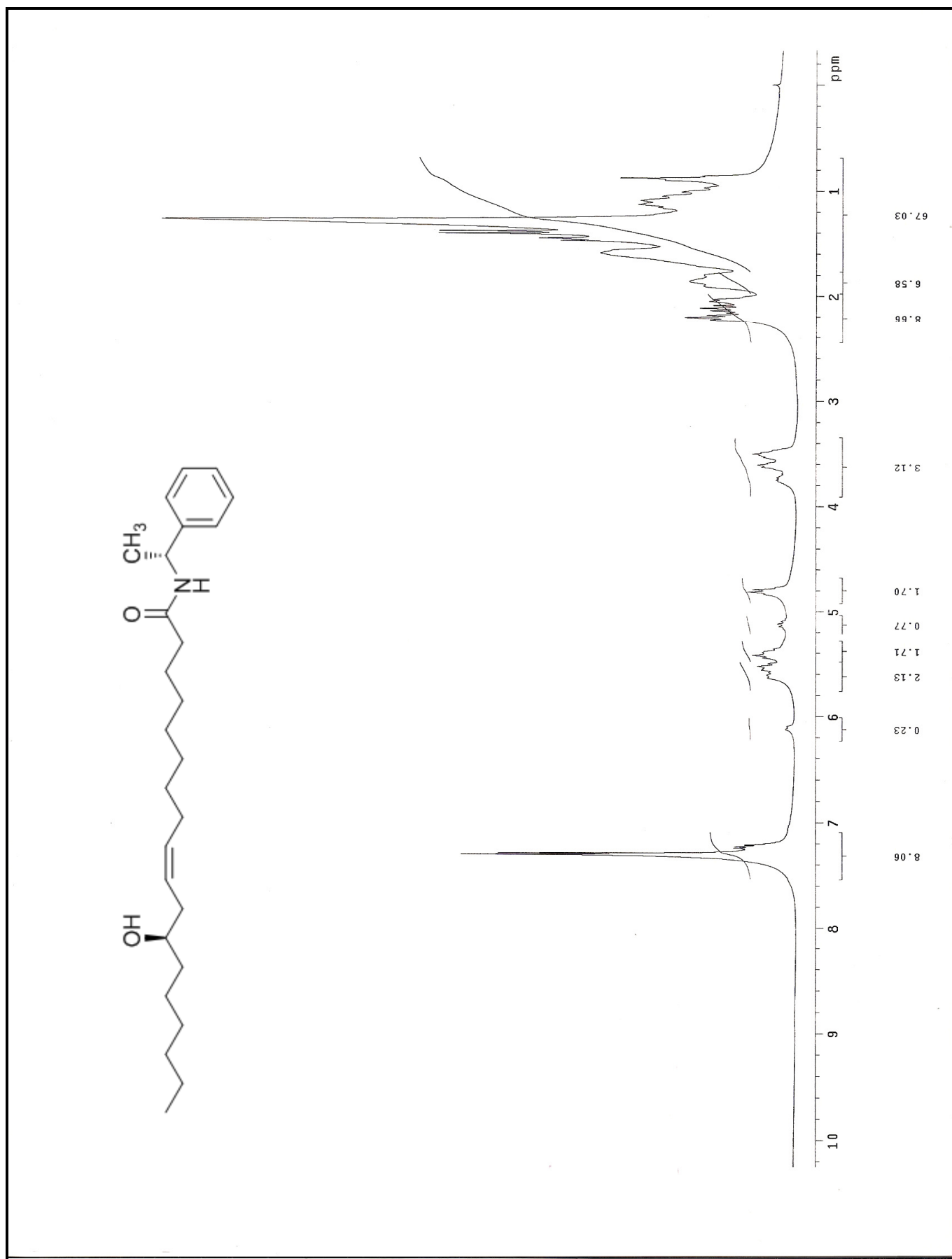
Espectro 45– RMN ^1\text{H} (300 Hz, \text{CDCl}_3 ) da ( R/R )- \alpha -metil- N -benzil-12-hidróxi-9- Z -octadecenamida (67d).
