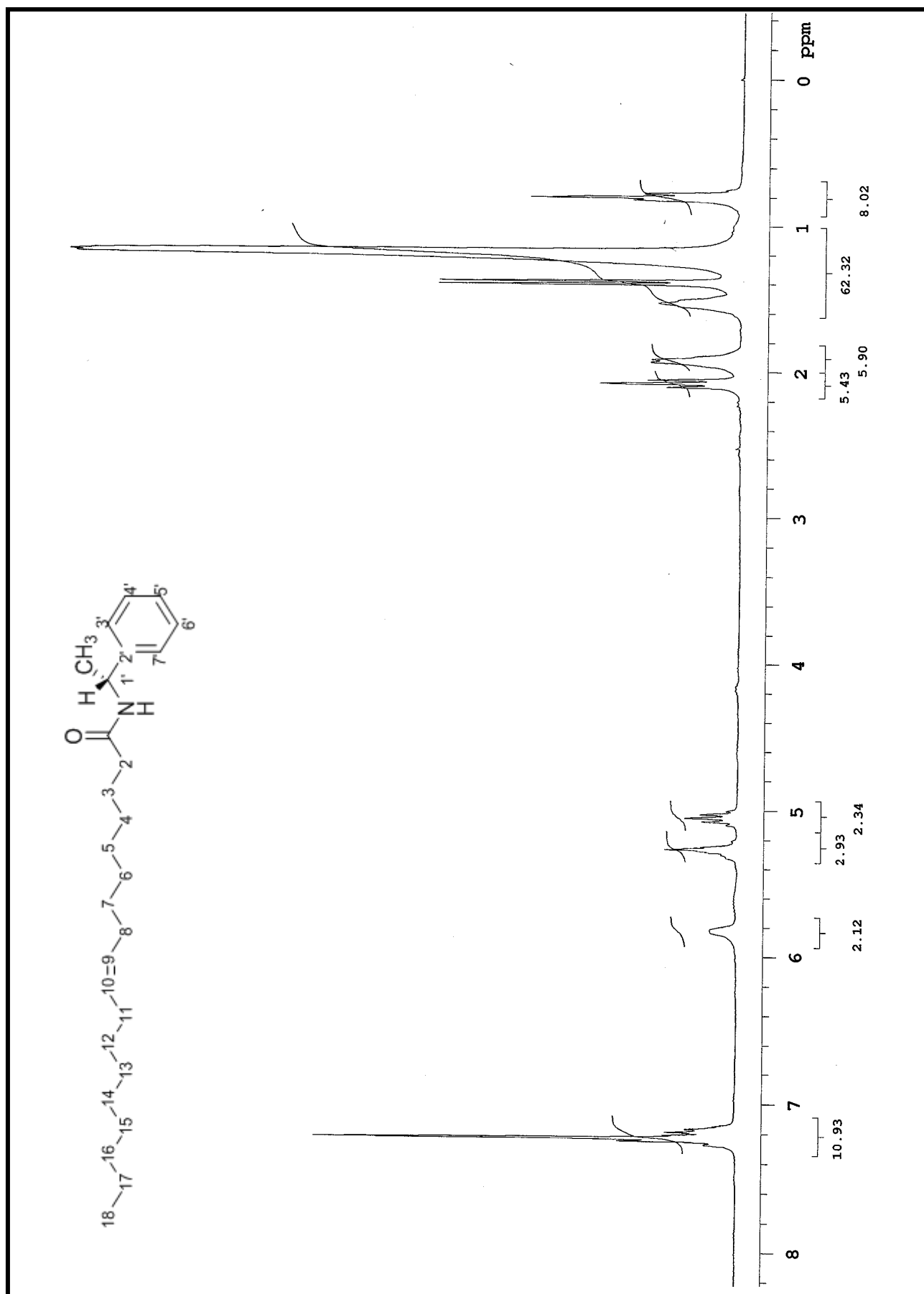
Figura 22 - Espectro RMN ^1\text{H} (300 MHz) para (R)-(+)-oleilmetilbenzilamida (R)-67c em \text{CDCl}_3
