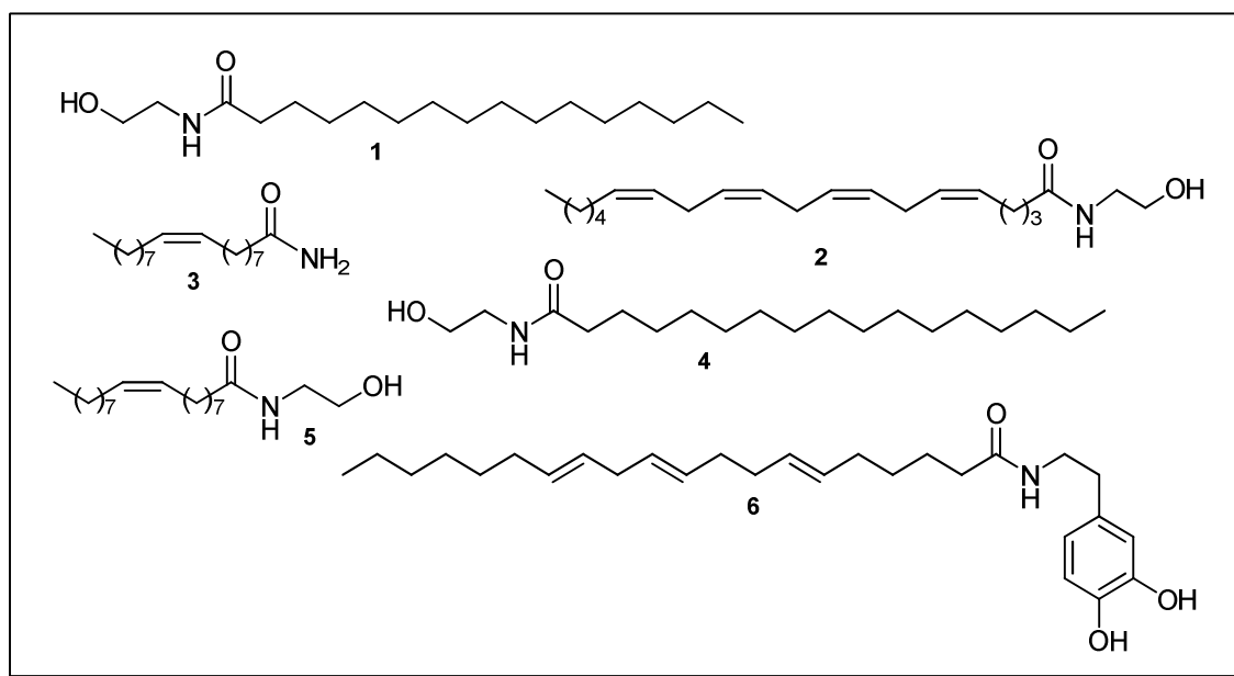
Figura 2 - Amidas graxas biologicamente ativas, N -palmitoiletanolamida ( 1 ), anandamida ( 2 ), cis -oleamida ( 3 ), N -esteariletanolamida ( 4 ), oleiletanolamida ( 5 ), dopamida graxa ( 6 ).
