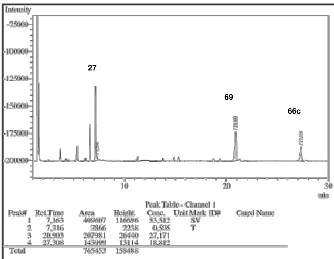
Figura 10 - Cromatograma bruto reacional 66c pelo método B7
