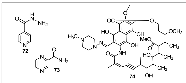
Figura 42 - Fármacos utilizados no tratamento de TB: isoniazida (INH, 72 ), pirazinamida (PZA, 73 ) e rifampicina ( 74 ).
