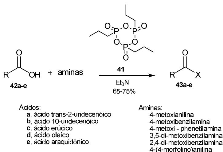
Esquema 16 - Síntese de amidas graxas utilizando PPAA.
