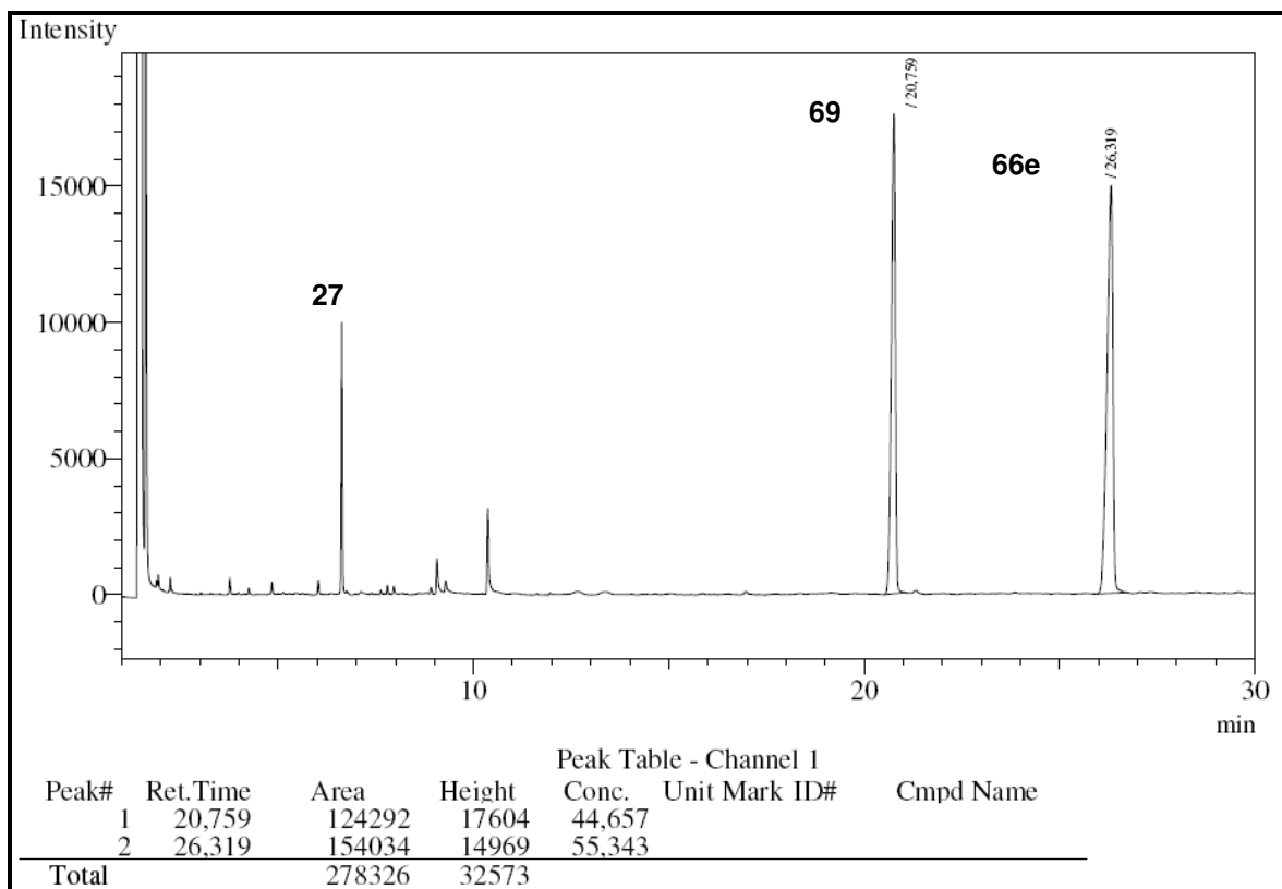
Figura 9 - Cromatograma bruto reacional de (R)- 66e pelo Método B3
