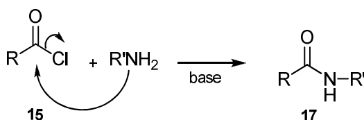
Esquema 5 - Aminólise de cloreto de acila.
