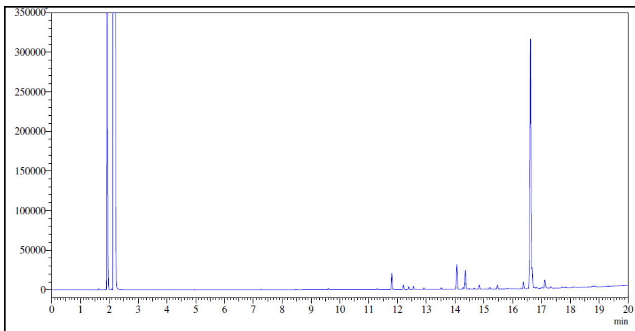
Cromatograma 3 – Oleato de metila 63c.
