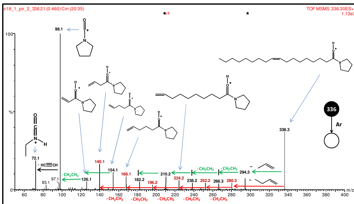
Figura 38 - Espectro de massas ESI-(+)-MS/MS da N -pirrolidil-9 Z -octadecenamida 75c .
