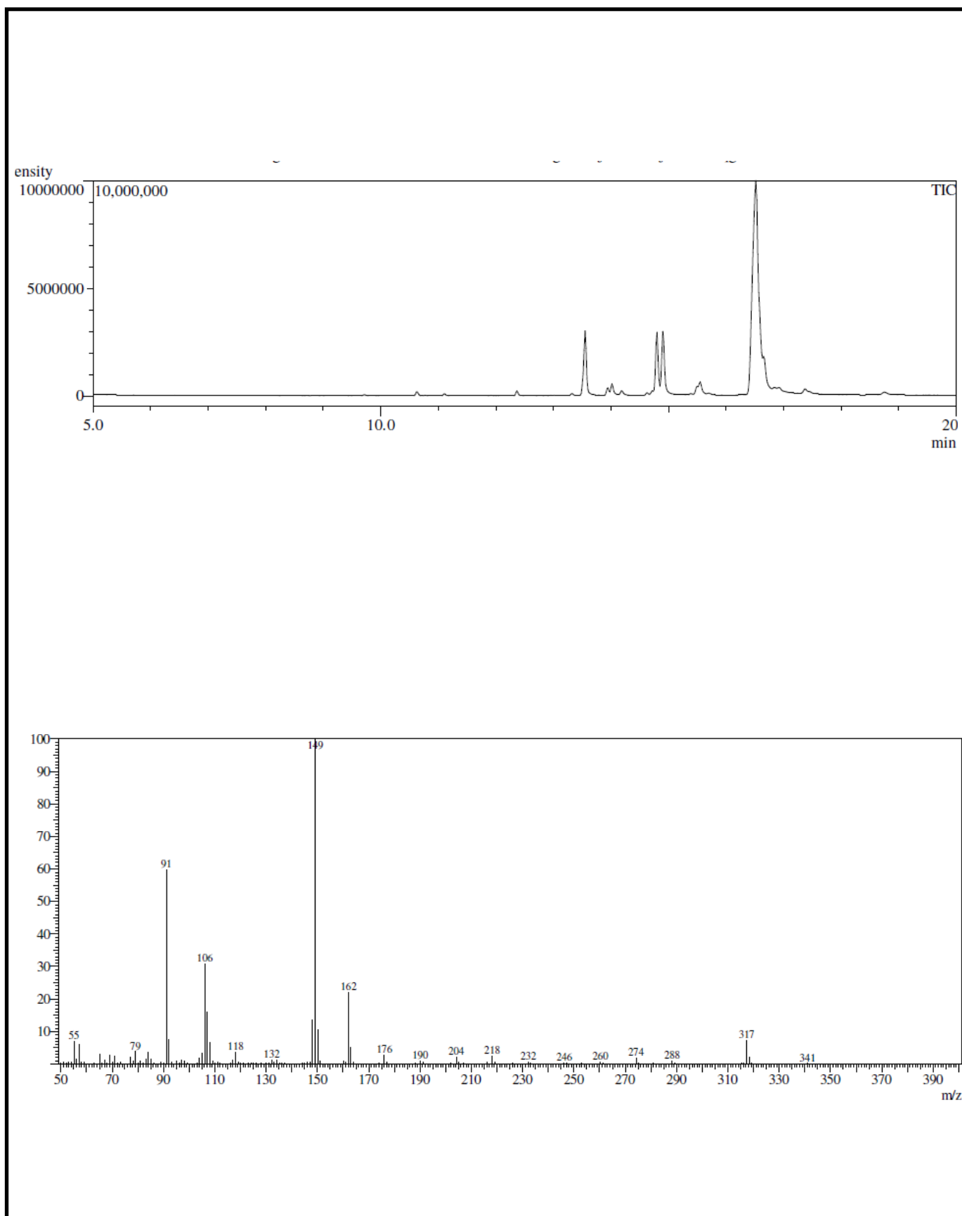
Espectro 17 – GC-MS da N -benzil-9- Z -octadecenamida ( 66c ).
