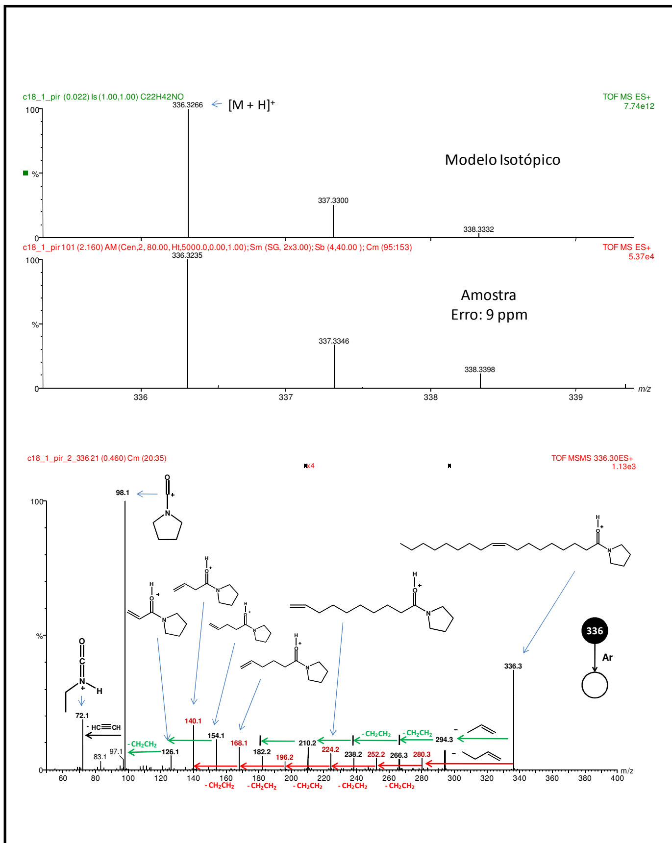
Espectro 58 – ESI-MS/MS da N -pirrolidil-9- Z -octadecenamida (75c).
