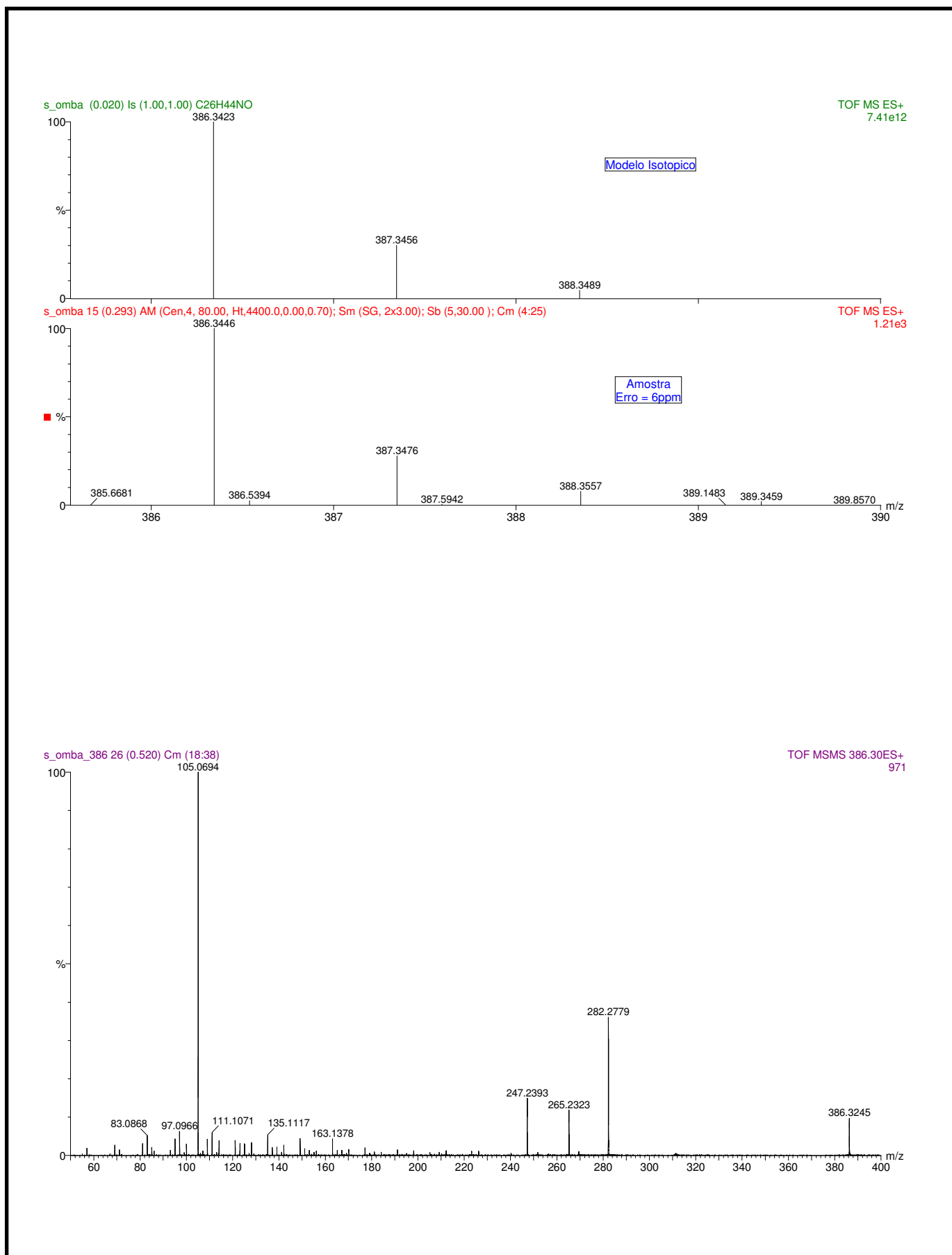
Espectro 41 – ESI-MS/MS da \alpha -metil-N-benzil-9-Z-octadecenamida ( 67c ).
