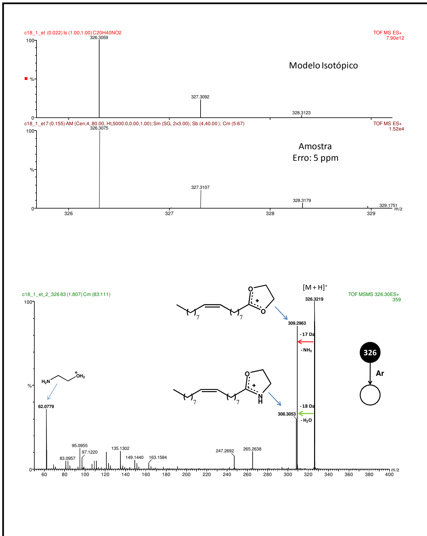
Espectro 68 – ESI-MS/MS da N -2-hidroxietyl-9- Z -octadecenamida ( 77c ).
