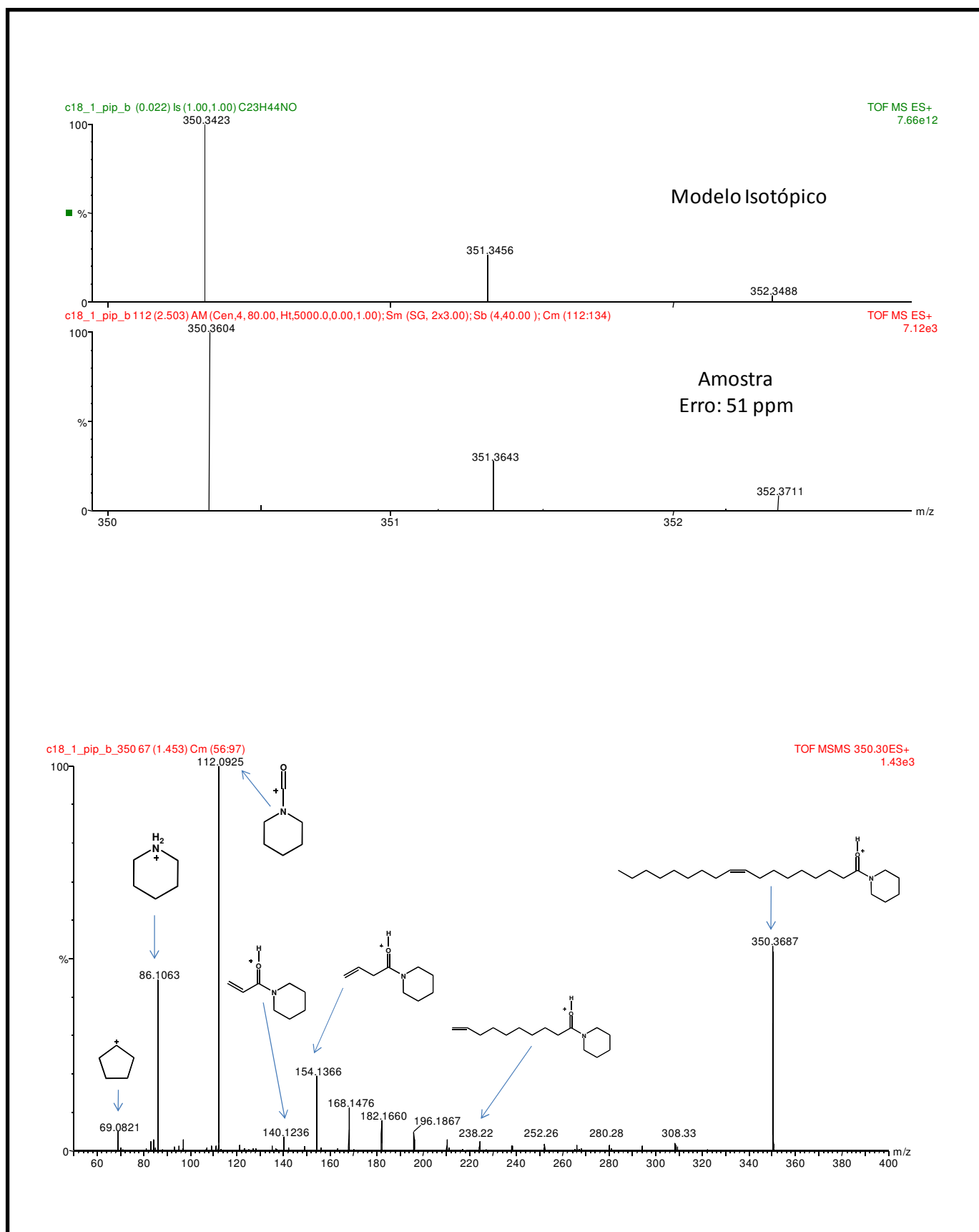
Espectro 75 – ESI-MS/MS da N -piperidinil-9- Z -octadecenamida (78c).
