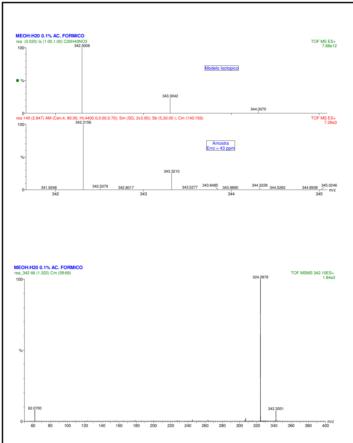
Espectro 70 – ESI-MS/MS da N-2-hidroxi-etil-12-hidroxi-9-Z-octadecenamida (77d).
