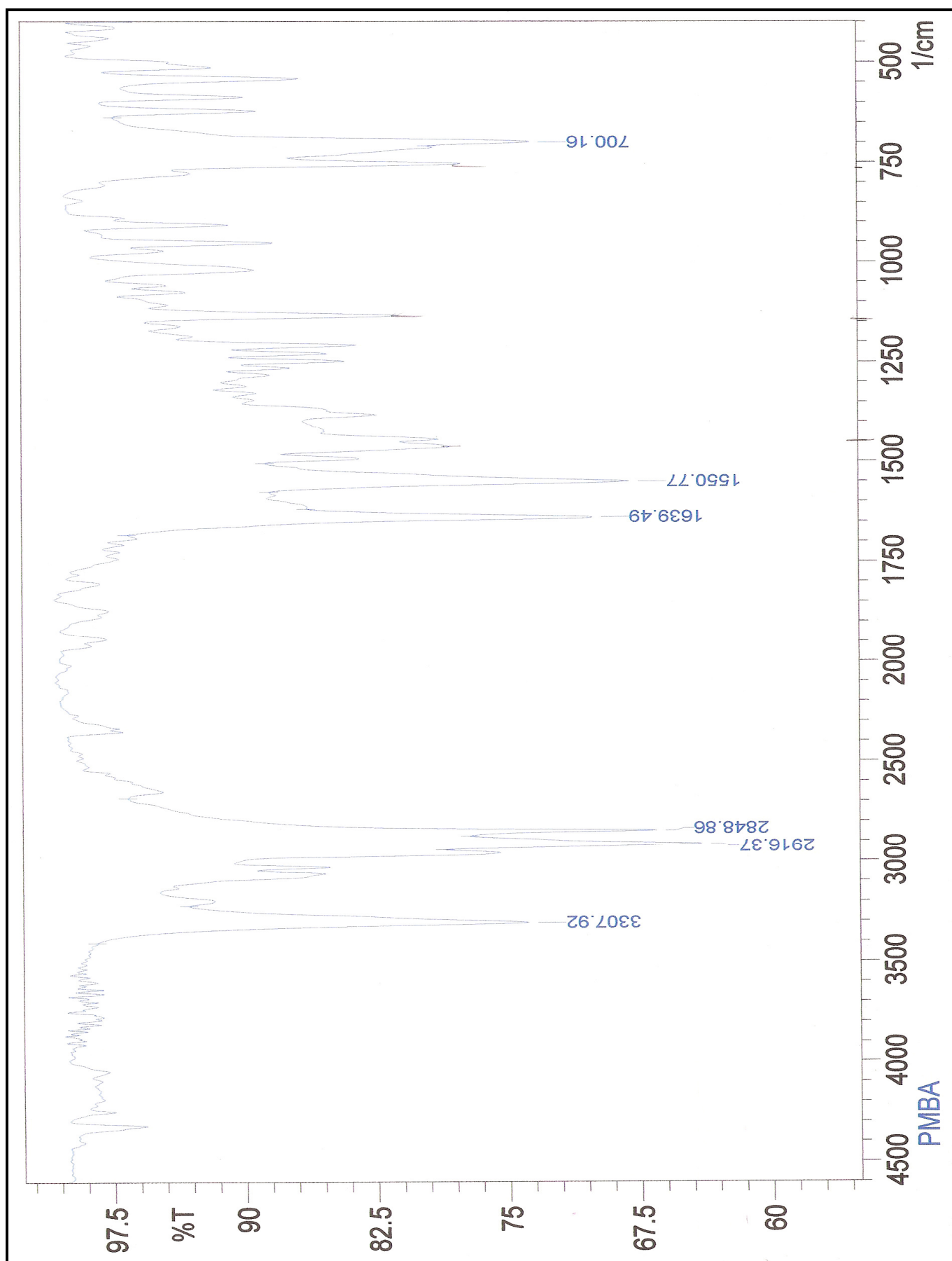
Espectro 29 – I.V. (Kbr) da \alpha -metil-N-benzil-hexadecanamida (67a).
