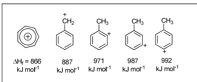
Figura 29 - Íon tropílio
