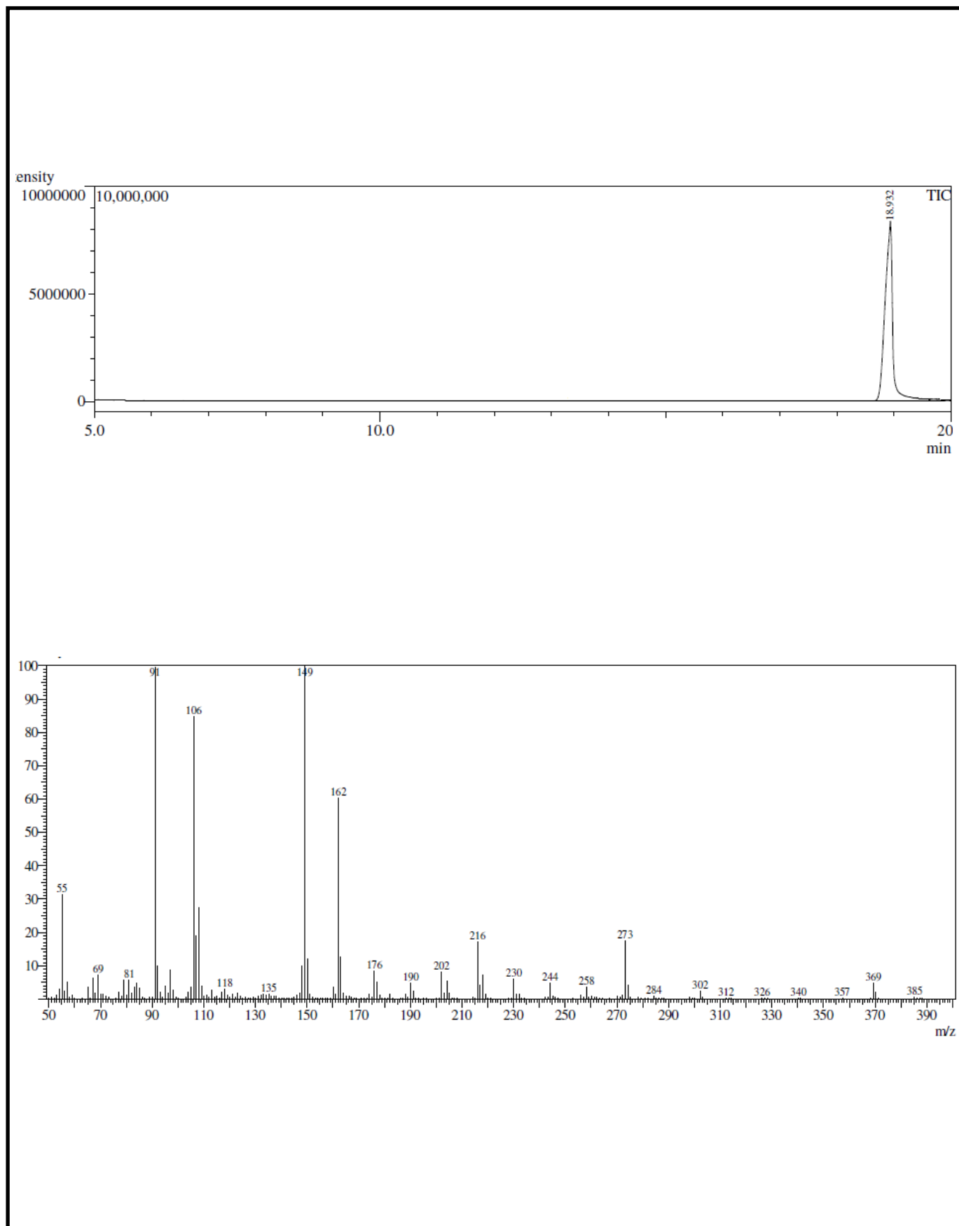
Espectro 22 – GC-MS da N -benzil-12-hidroxi-9- Z -octadecenamida ( 66d ).
