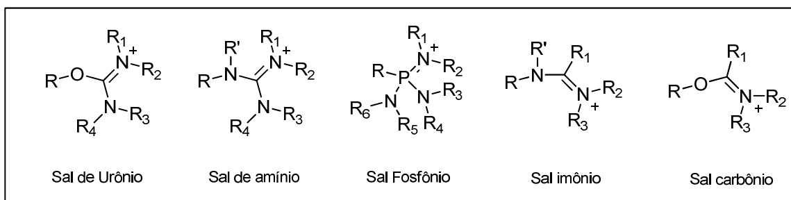
Figura 4 - Sais associados com reagentes baseados em HOBt 49 .
