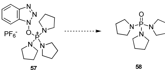
Figura 5 - PyBOP 57 e seu sub-produto 1,1',1''- fosforiltripirrolidina 58 .
