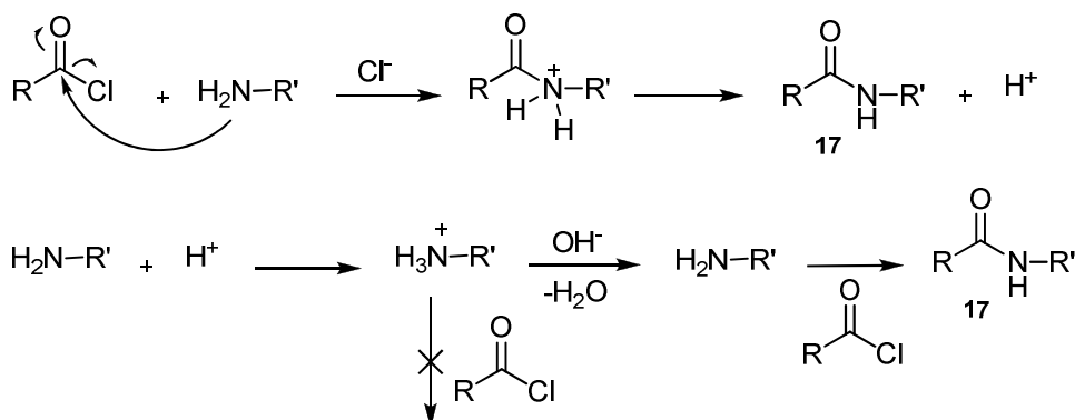
Esquema 6 - Síntese de amidas nas condições Schotten-Baumann.
