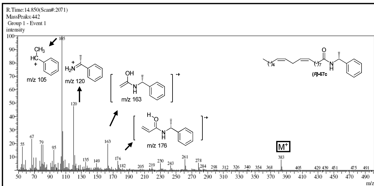
Figura 32 - Espectro de massas (GC-MS) da N -benzil-9 Z ,10 Z -octadecenamida ( R )- 67c .
