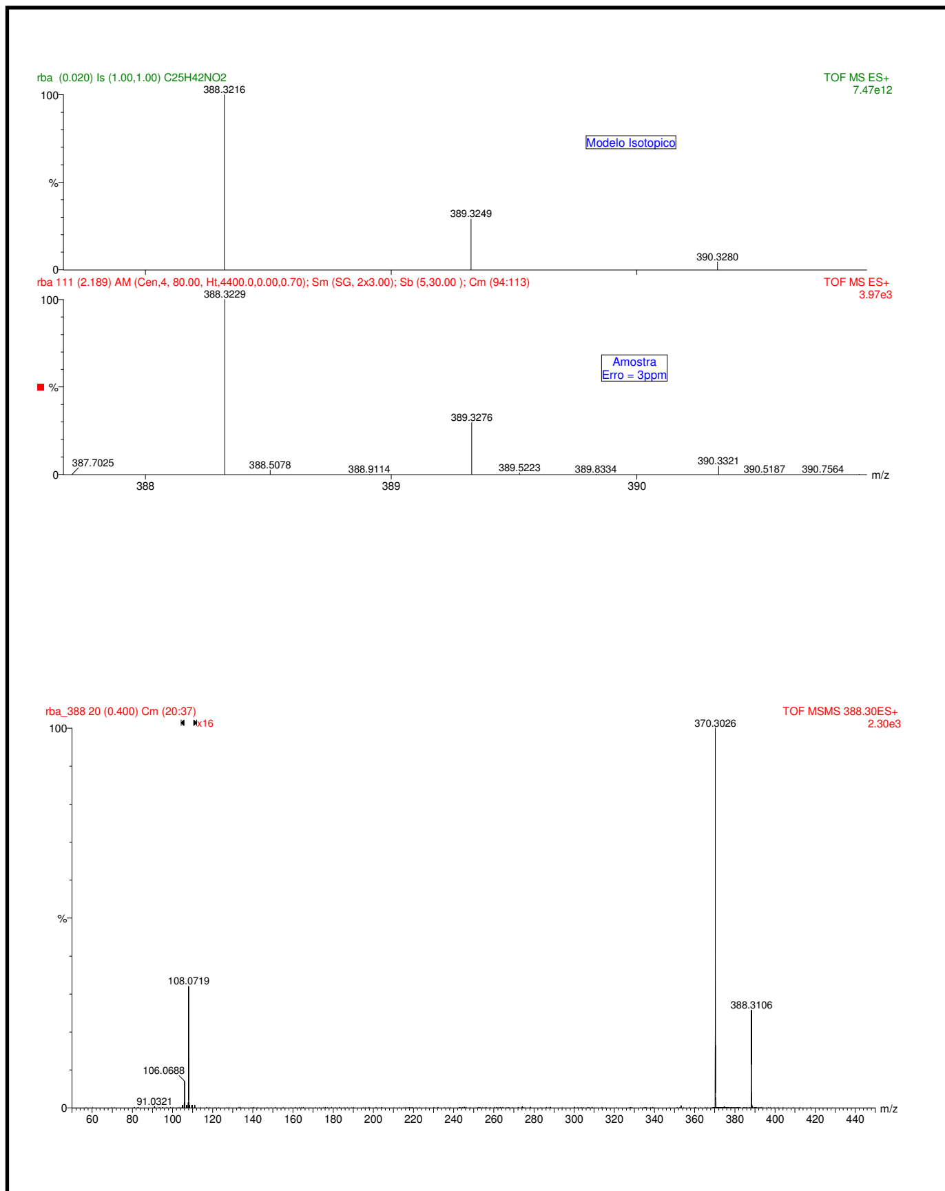
Espectro 23 – ESI-MS/MS da N -benzil-12-hidroxi-9- Z -octadecenamida ( 66d ).
