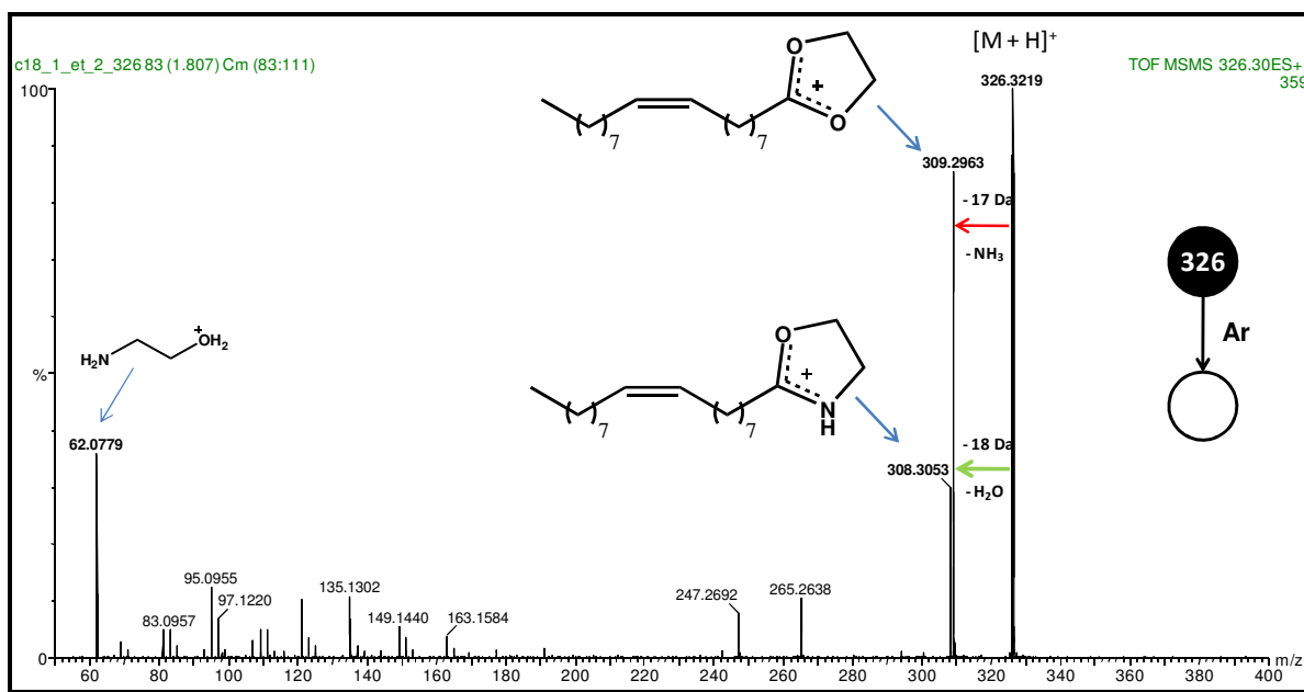
Figura 36 – Espectro ESI-(+)-MS/MS da N -hidroxietil-9- Z -octadecenamida ( 77c ).
