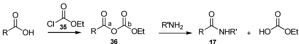
Esquema 14 - Síntese de amidas a partir de anidrido etóxicarbonílico (36).
