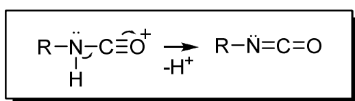
Figura 41 – Perda de \text{H}^+ do íon acílio para formação de espécie neutra.
