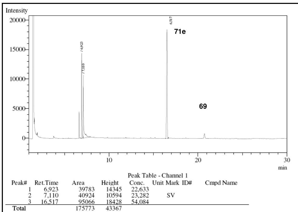
Figura 13 - Cromatograma bruto reacional da Linoleilpirrolidilamida 71e
