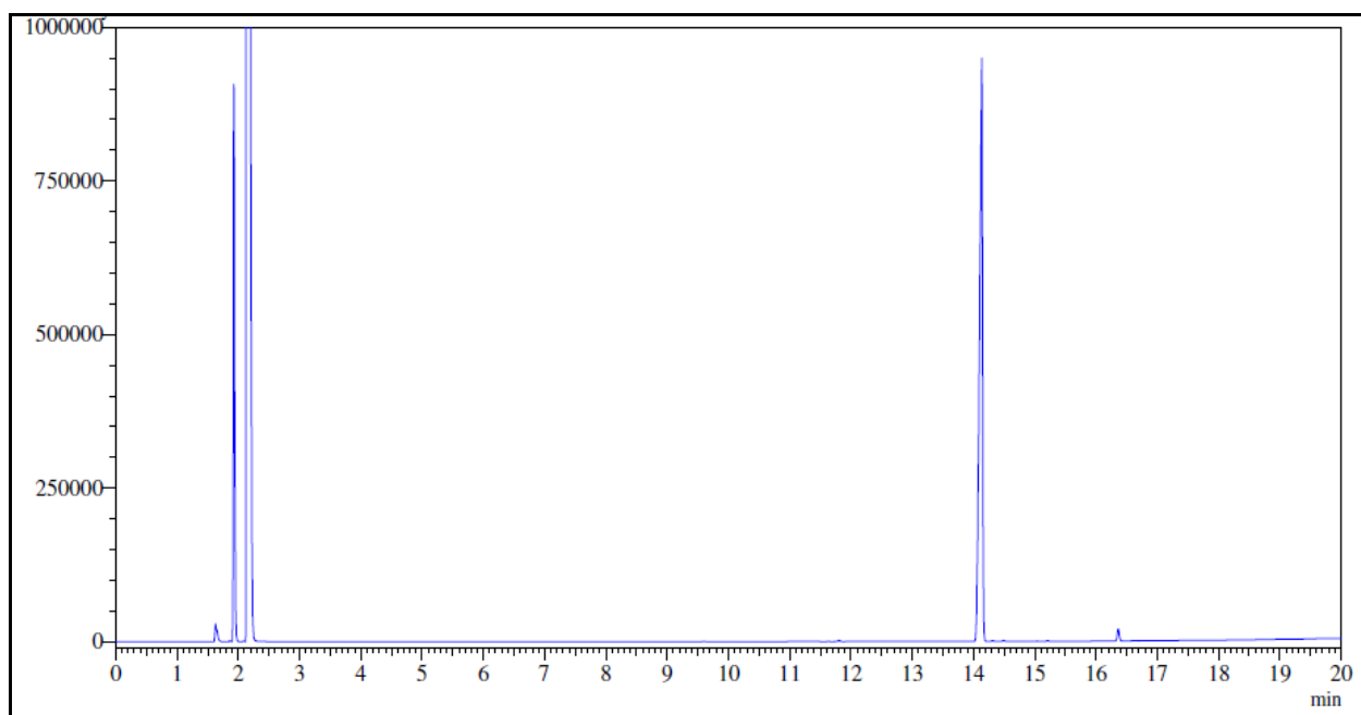
Cromatograma 1 – Palmitato de metila 63a.
