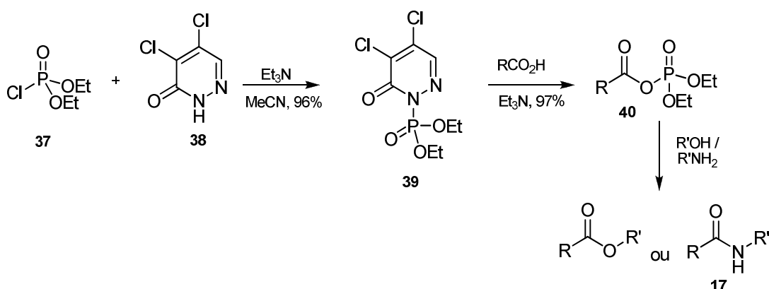
Esquema 15 - Síntese de amidas e ésteres a partir dietilclorofosfato (37).
