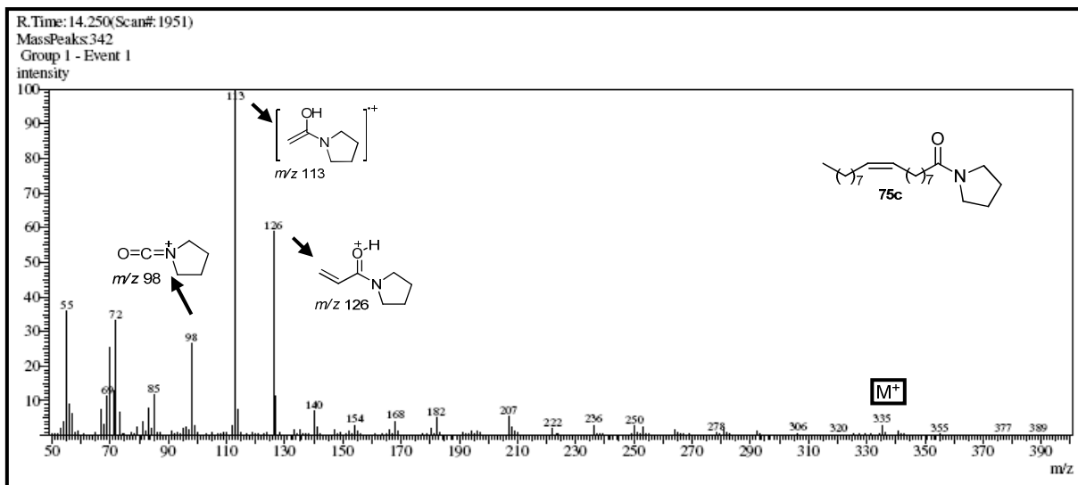
Figura 37 - Espectro de massas(GC-MS) da N -pirrolidil-9 Z -octadecenamida 75c .
