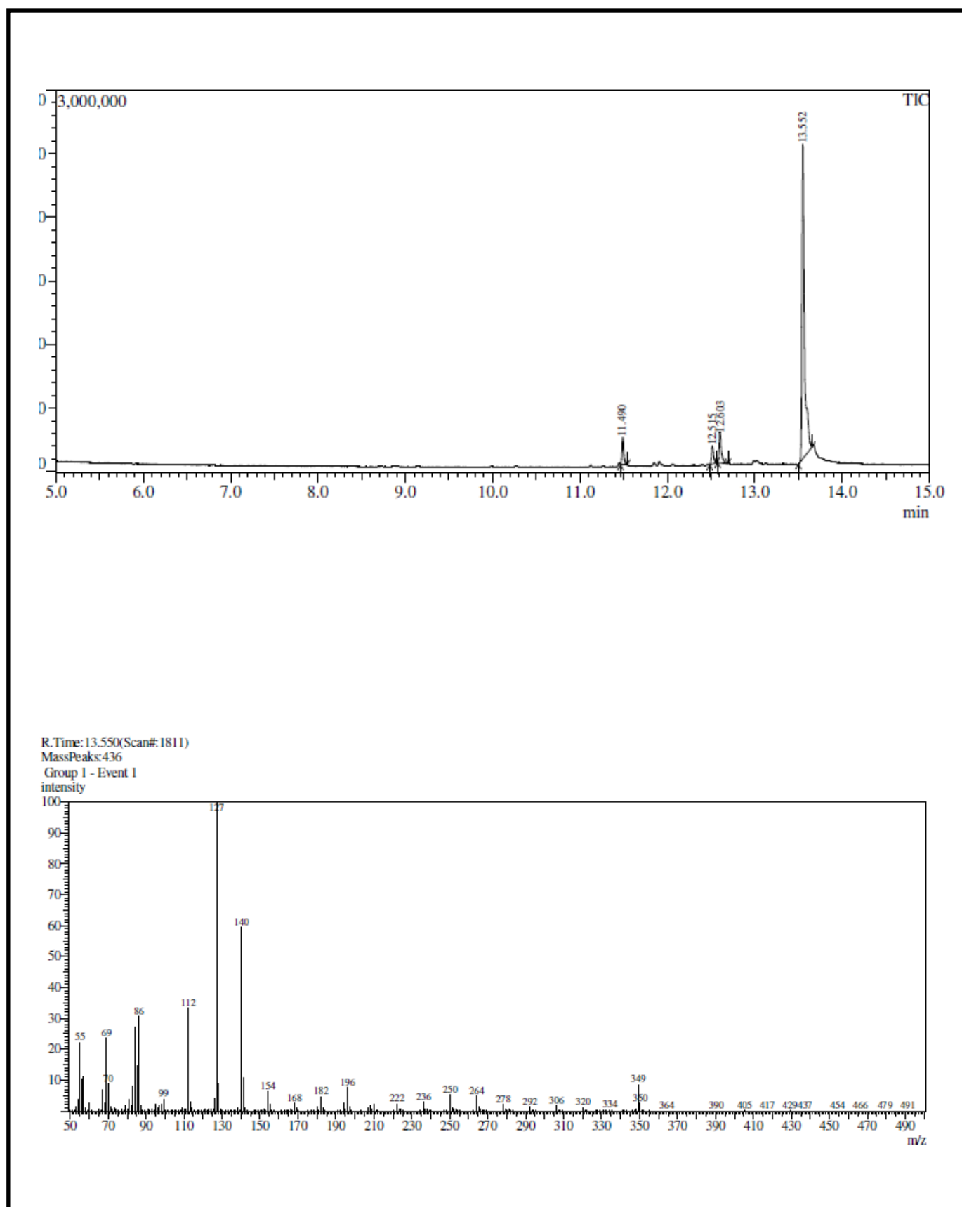
Espectro 74 – GC-MS (70eV) da N -piperidinil-9- Z -octadecenamida ( 78c ).
