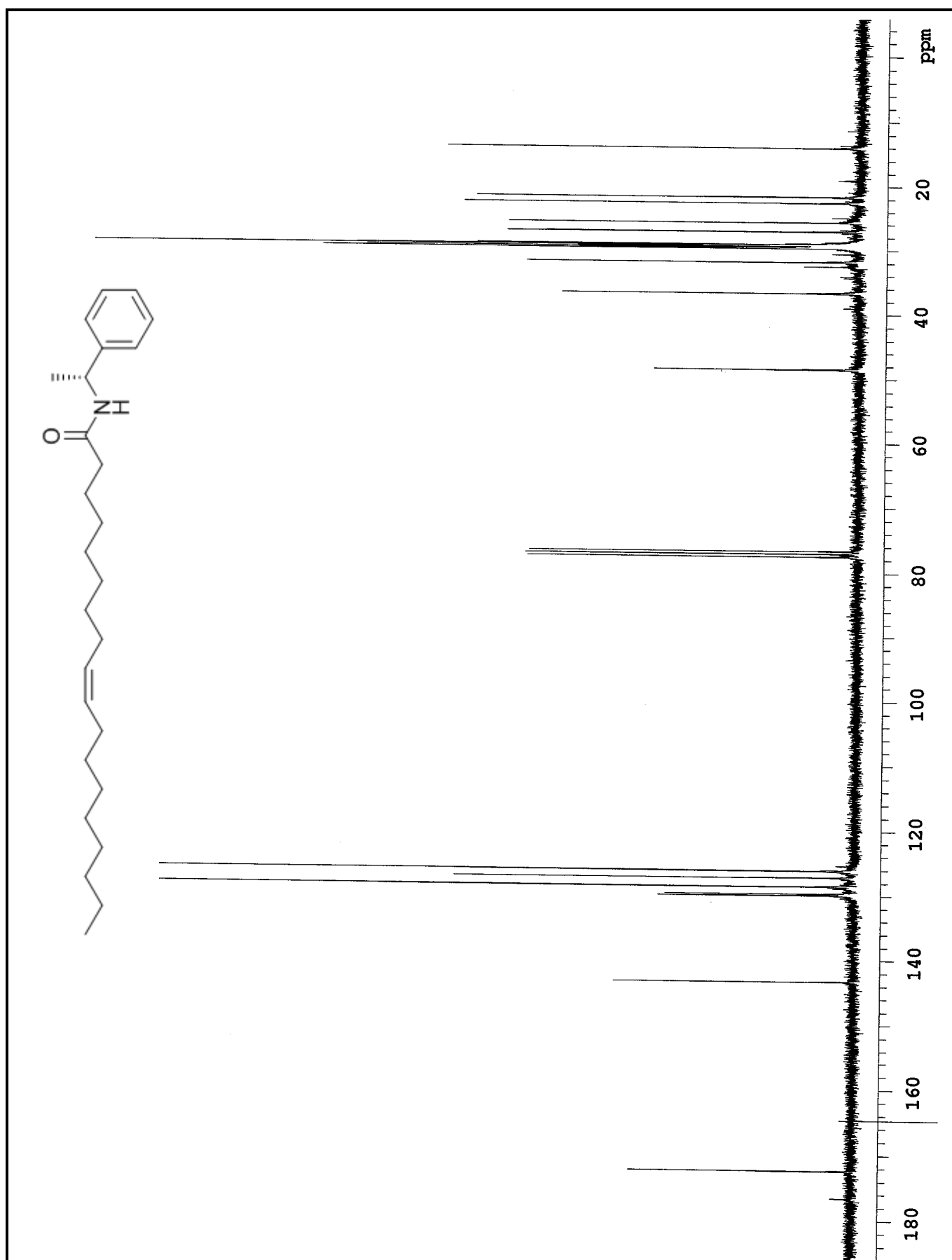
Espectro 39 – RMN ^{13}\text{C} (75 Hz, \text{CDCl}_3 ) da \alpha -metil- N -benzil-9- Z -octadecenamida ( 67c ).
