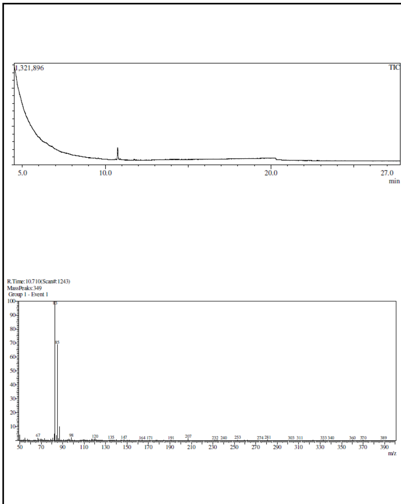
Espectro 65 – GC-MS (70 eV) da N -2-hidroxiethylhexadecanamida ( 77a ).
