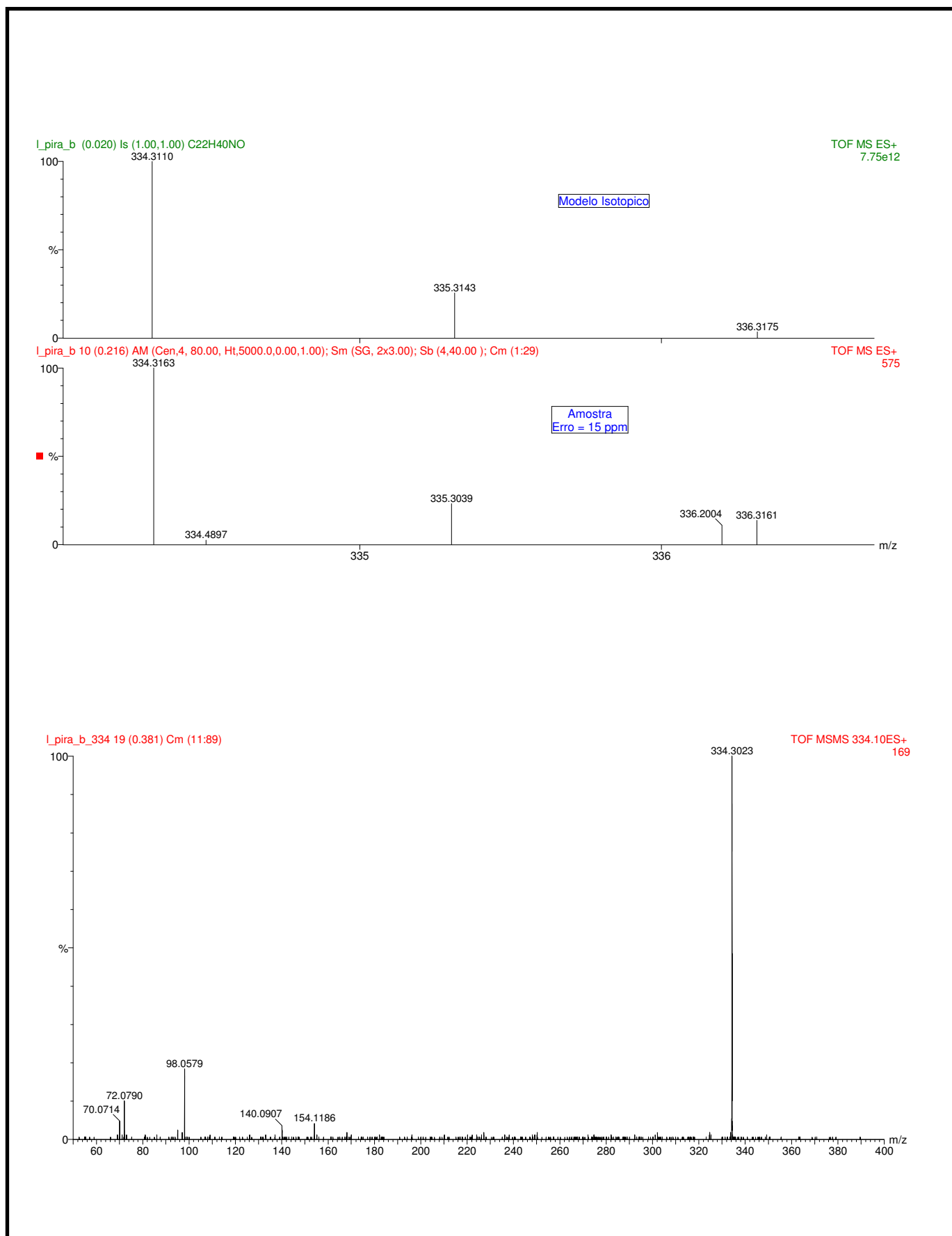
Espectro 54 – ESI-MS/MS da N -pirrolidil-9,12- Z -octadecenamida ( 71e ).
