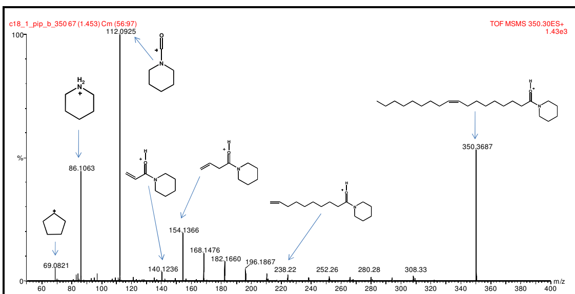
Figura 40 - Espectro de massas ESI(+)-MS/MS da N -piperidil-9 Z -octadecenamida 77c .
