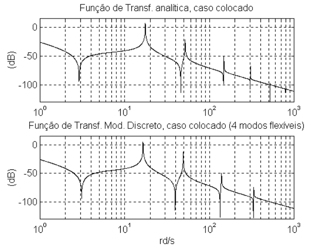
Figura 6: Funções de Transferência Analítica e do Modelo Discreto com 4 modos flexíveis (caso colocado-4af), sendo negligenciados os torques de atrito do Modelo Discreto.
